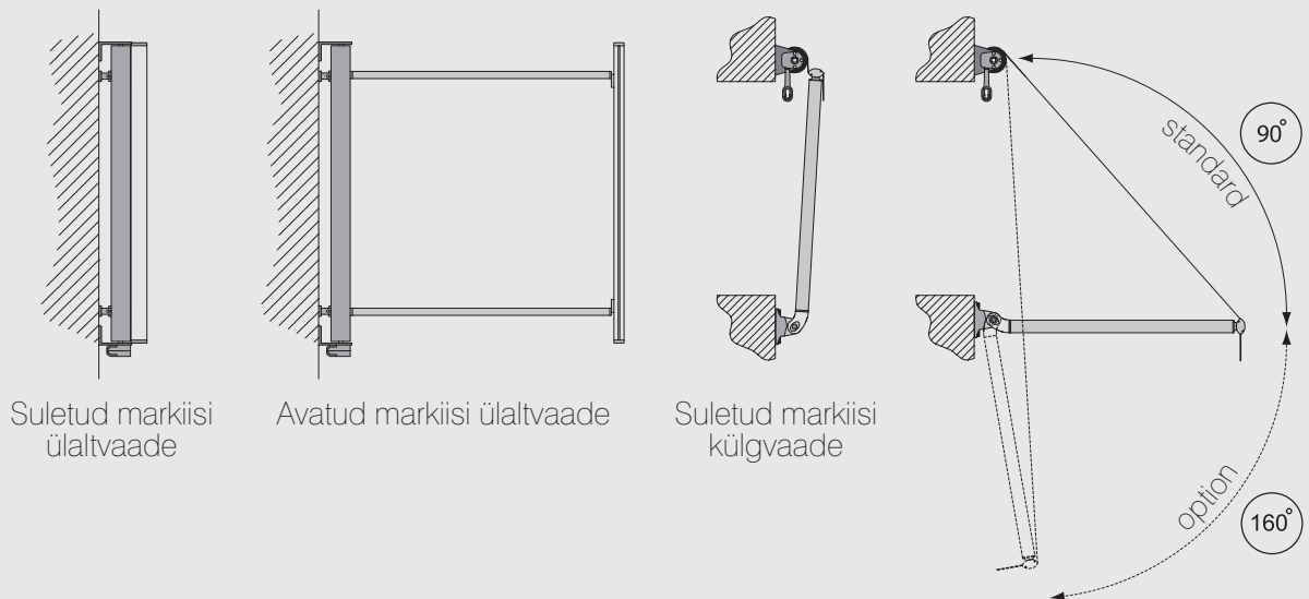
Avatud markiisi külgsaade. Üle 90° kaldenurga puhul tuleb kanga eest juurde maksta
